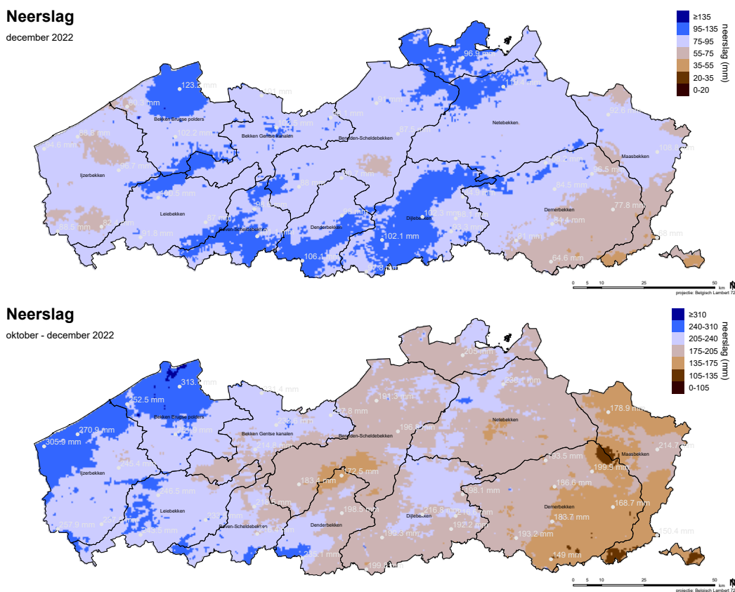
Figuur 1: Neerslagtotalen voor de voorbije maand, resp. voorbije 3 maanden op basis van het Vlaamse neerslagdarcosmposit (achtergrond) en VMM-pluviometernetwerk (punten).
