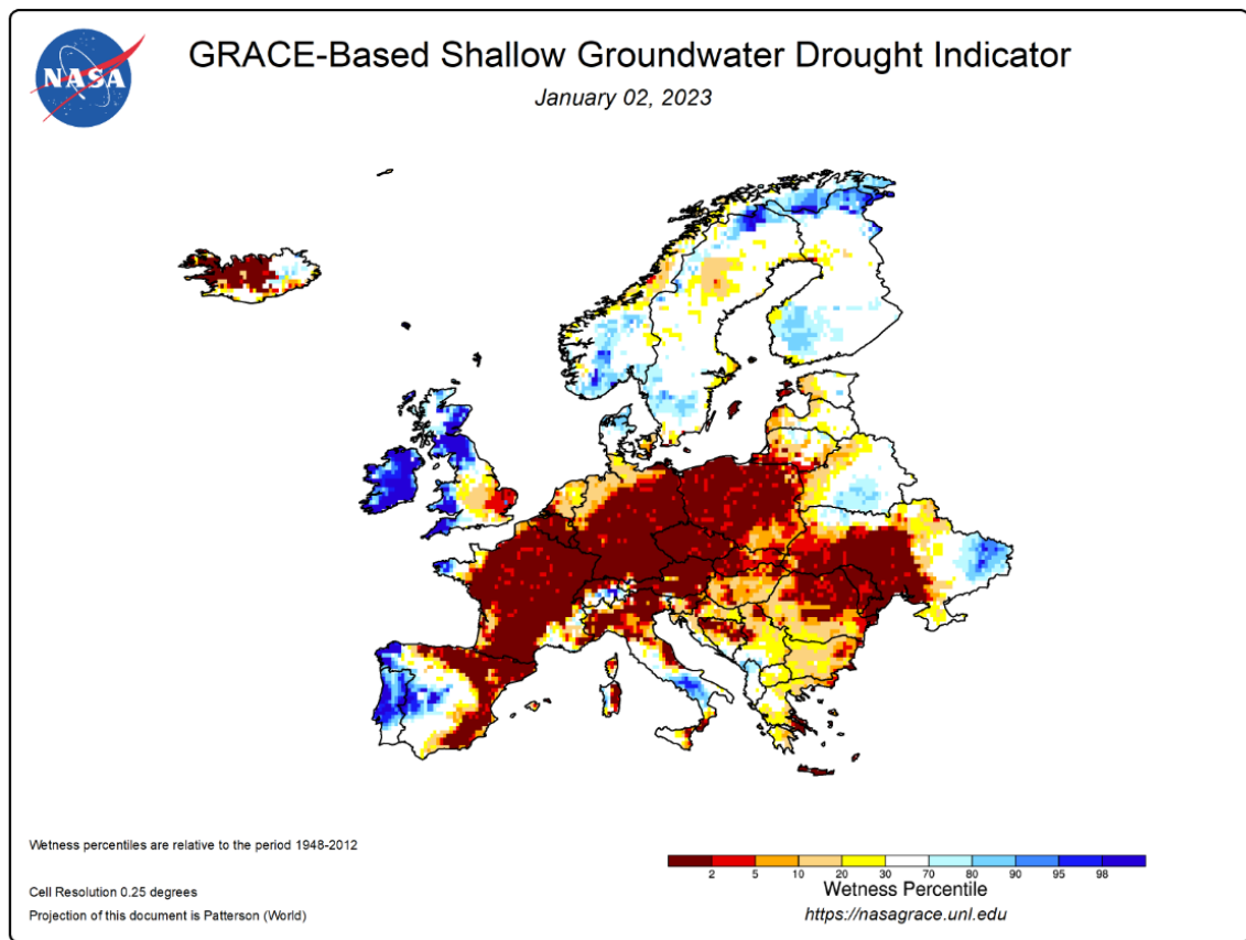
Figuur 9: Oppervlakkige grondwaterdroogte-indicator van NASA voor Europa op 2/01/2023, gebaseerd op GRACE-FO Data (beschikbaar op https://nasagrace.unl.edu , geconsulteerd op 5/01/2023)
