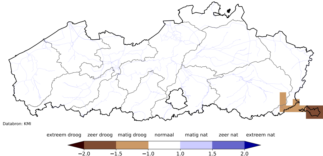
SPI3 waarneming voor 2023-01-02
