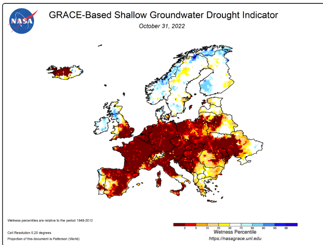
Figuur 9: Oppervlakkige grondwaterdroogte-indicator van NASA voor Europa op 31/10/2022, gebaseerd op GRACE-FO Data (beschikbaar op https://nasagrace.unl.edu , geconsulteerd op 7/11/2022)
