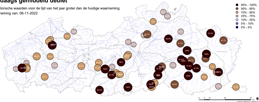
Figuur 14: 14-daags gemiddeld debiet als percentiel (overschrijding) van de historische waarden voor dezelfde periode van het jaar.
